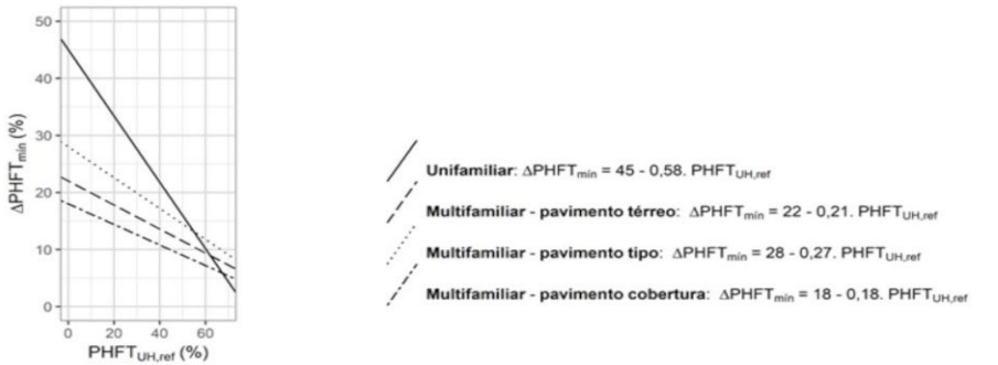
Figura 8.1. Ábaco e equações para a obtenção do ΔPHFTmín quando o PHFTUH,ref for menor ou igual a 70%
