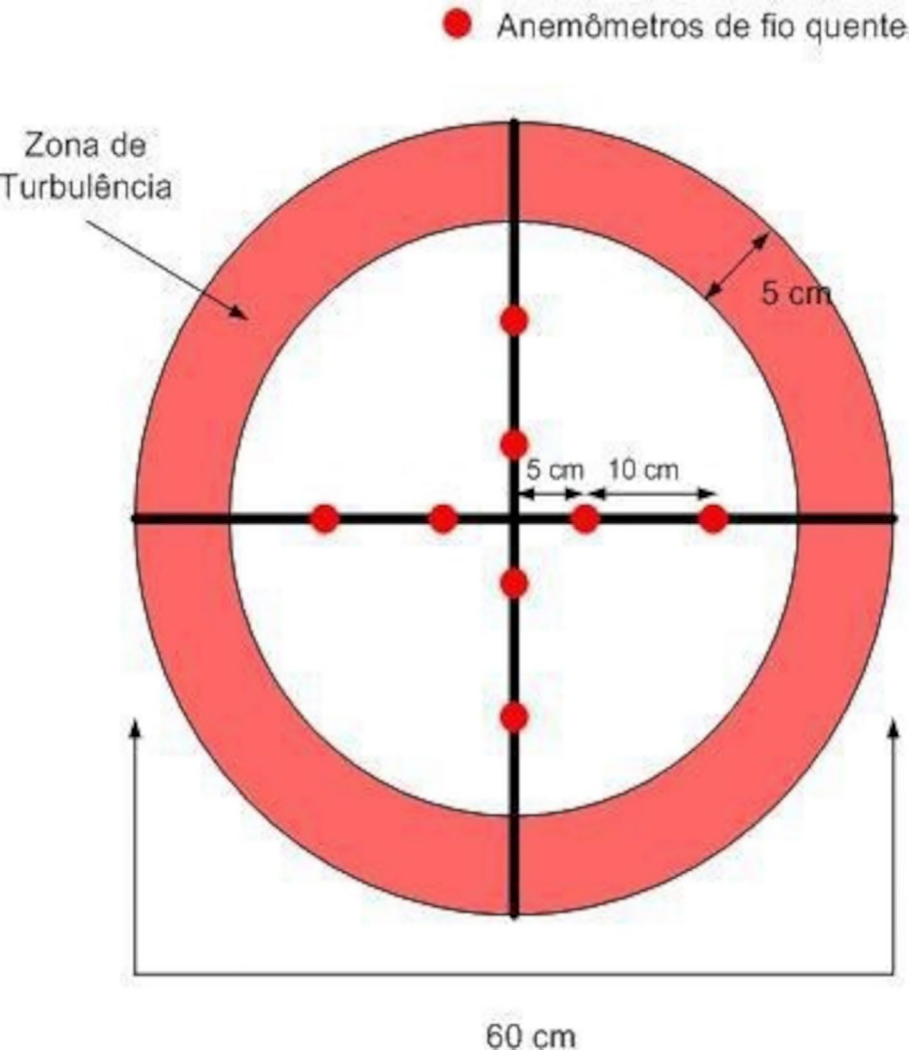
Figura 2 - Posição dos anemômetros no plano do duto
