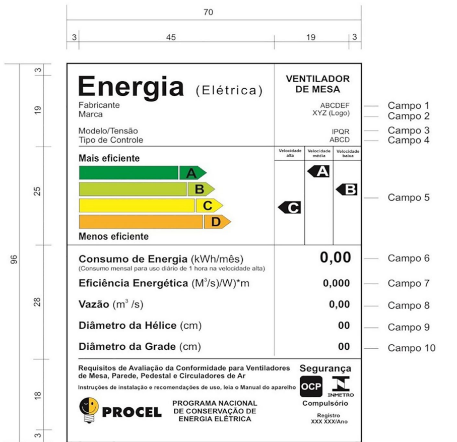
Figura II.3 - modelo para 3 (três) velocidades
