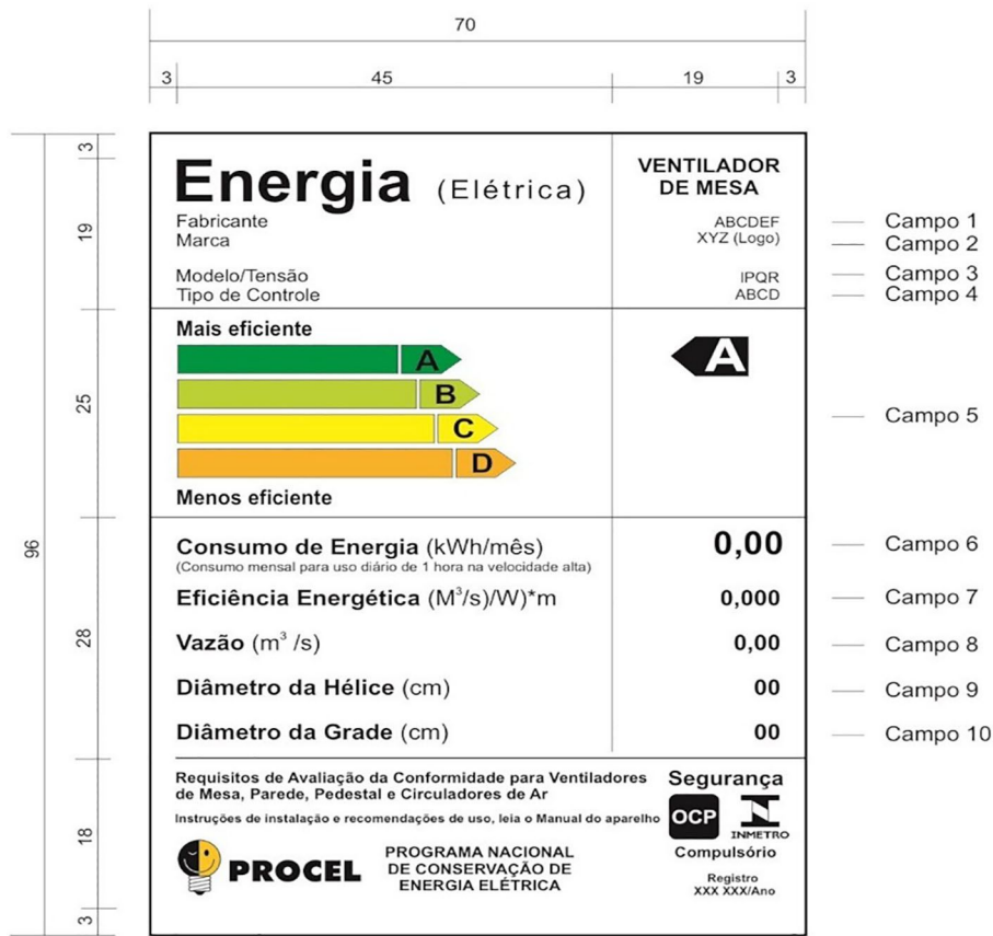
Figura II.2 - modelo para 1 (uma) velocidade
