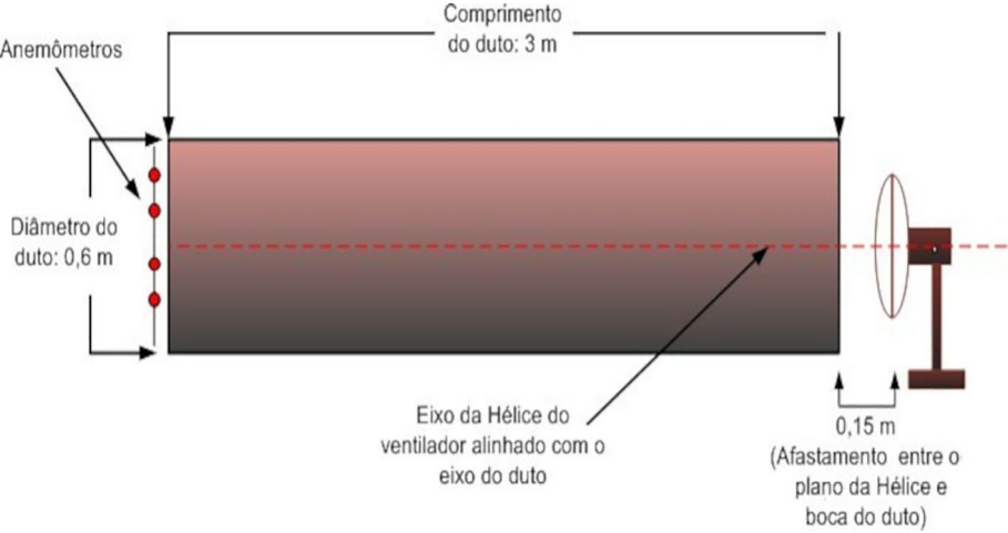
Figura 1 - Aparato de medição
