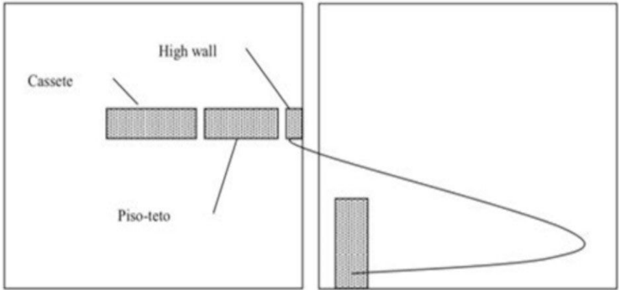
Figura B.1. Ilustração da instalação de condicionador de ar do tipo split em calorímetro - Vista frontal
