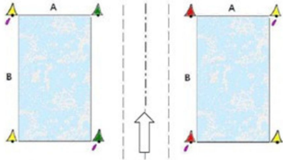
Duas áreas aquícolas retangulares, com sinais luminosos nas diagonais e com um canal de navegação entre elas. A seta branca indica a direção convencional de balizamento escolhida.
