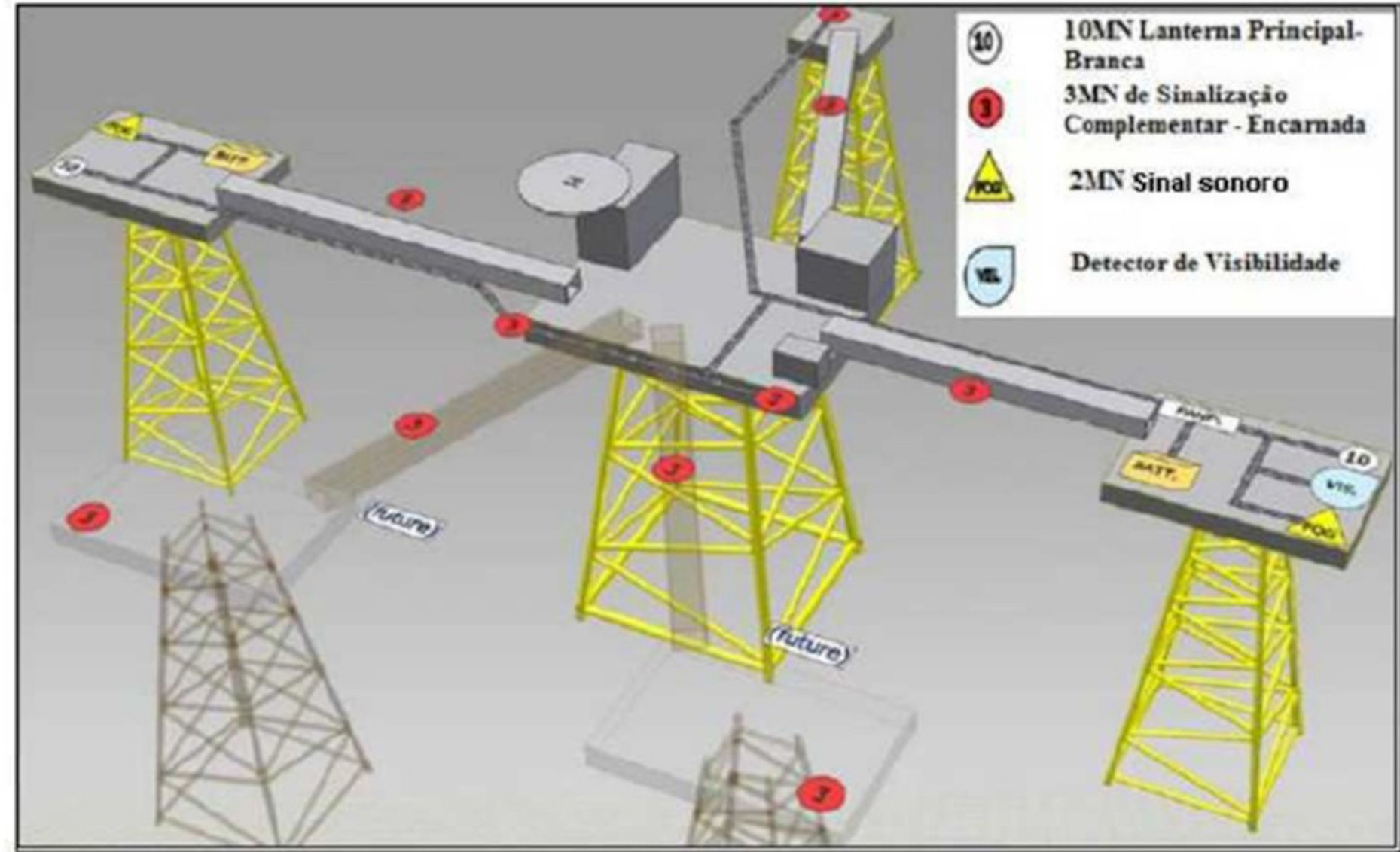
Sinalização de Estruturas Offshore. Fonte: Modificado da publicação IALA Recommendation O-139 –The Marking of Man-made Offshore Structures.
