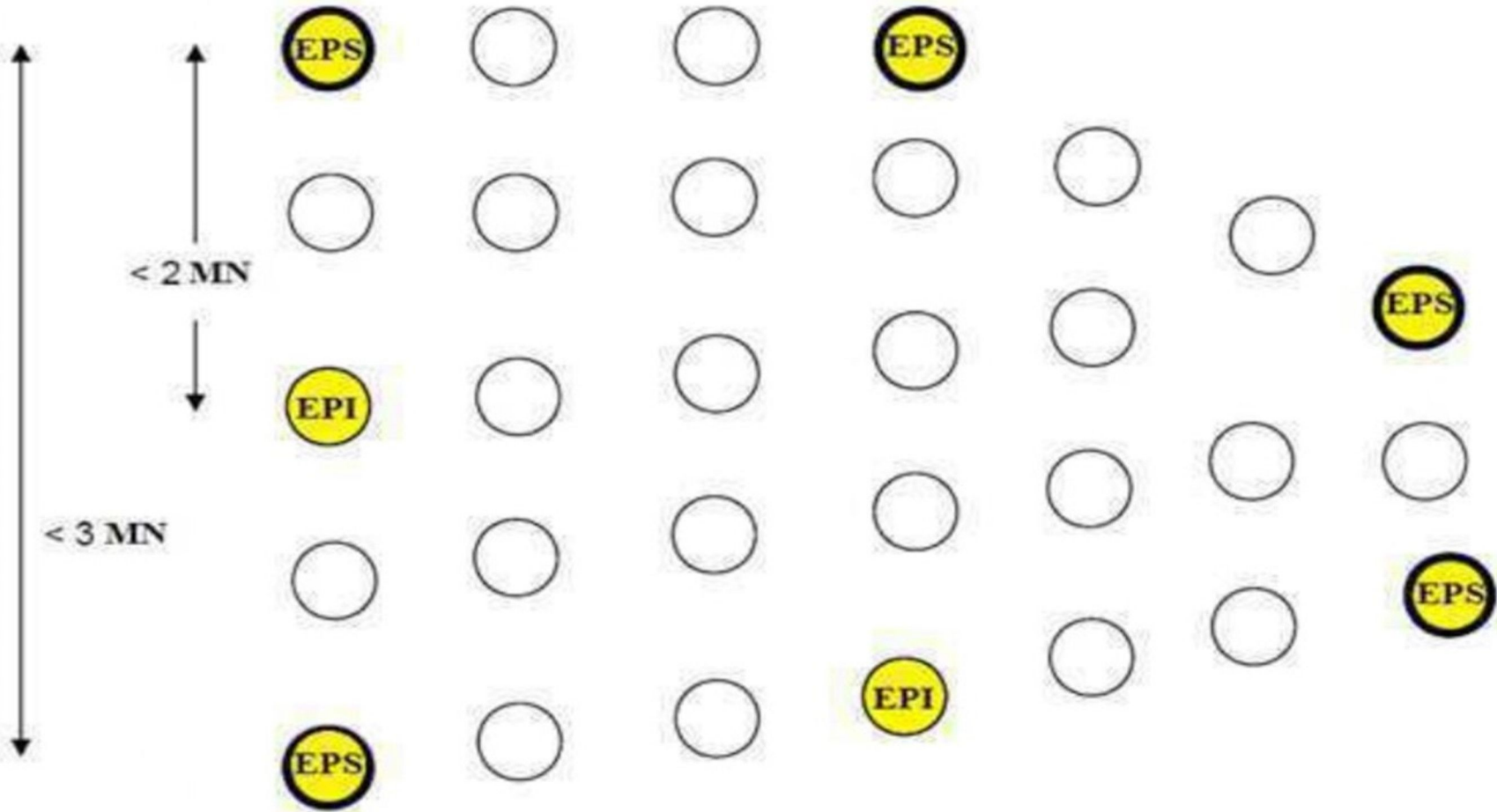
Sinalização simplificada de um Parque Eólico Offshore. Fonte: Modificado da Recomendação da IALA O-139, "The Marking of Man-made Offshore Structures".
