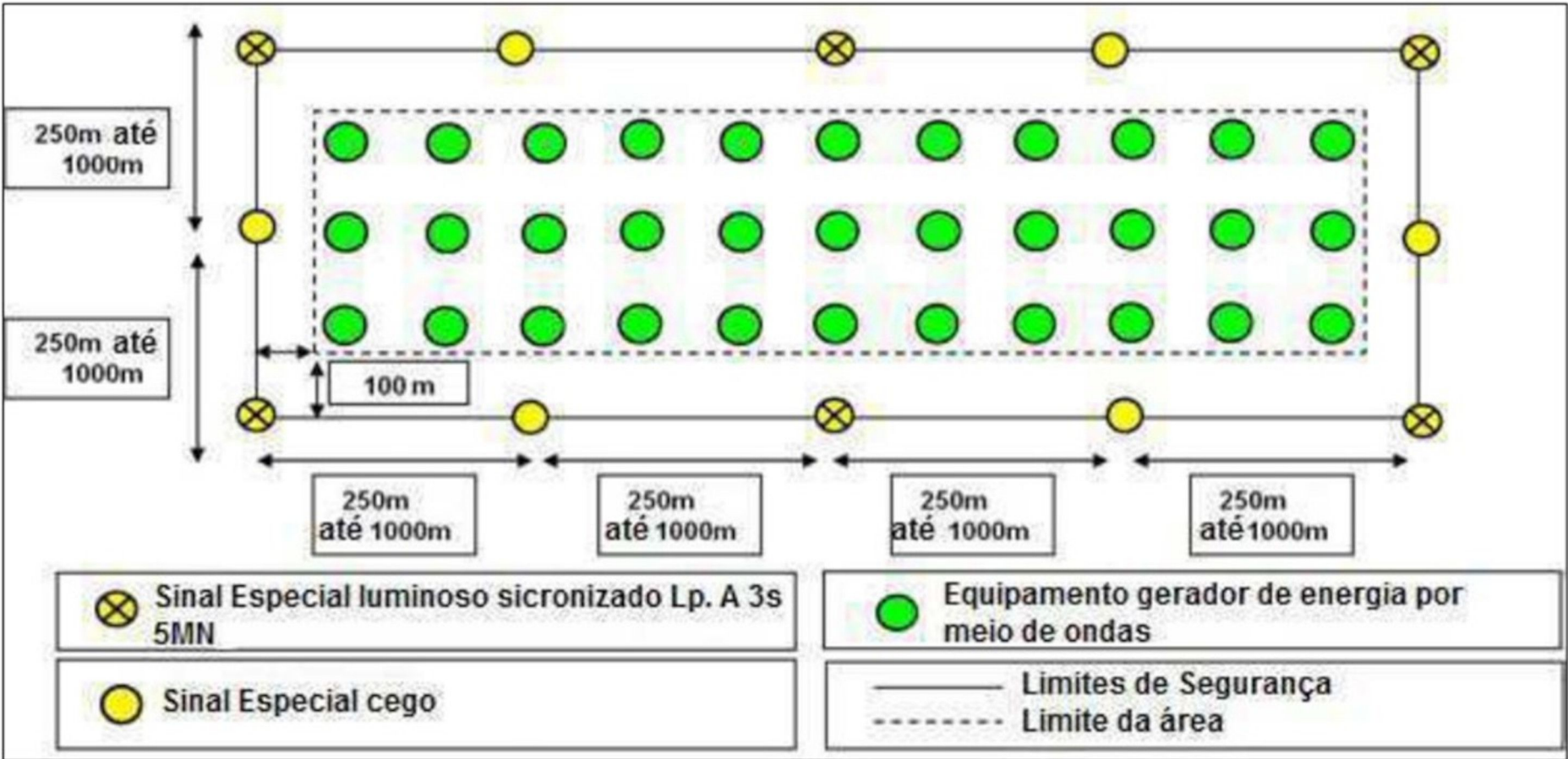
Sinalização de equipamentos. Fonte: Recomendação da IALA O-139, “The Marking of Man-made Offshore Structures”.
