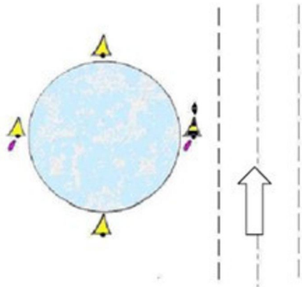
Balizamento de um canal de navegação com sinal Cardinal Leste. Neste arranjo, a direção convencional de balizamento é do Sul para o Norte.
