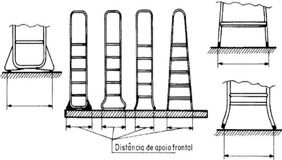
Figura 3 - Distância de Apoio Frontal e Traseiro
