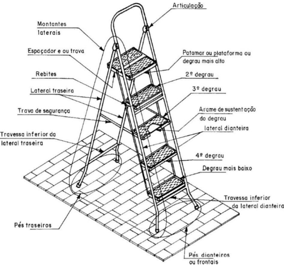
Figura 1 - Componentes da Escada
