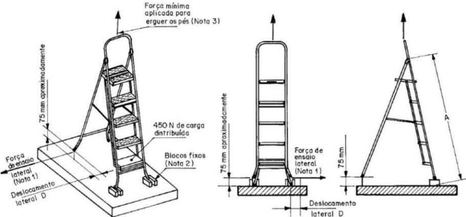
Figura 8 - Ensaio da Estrutura
