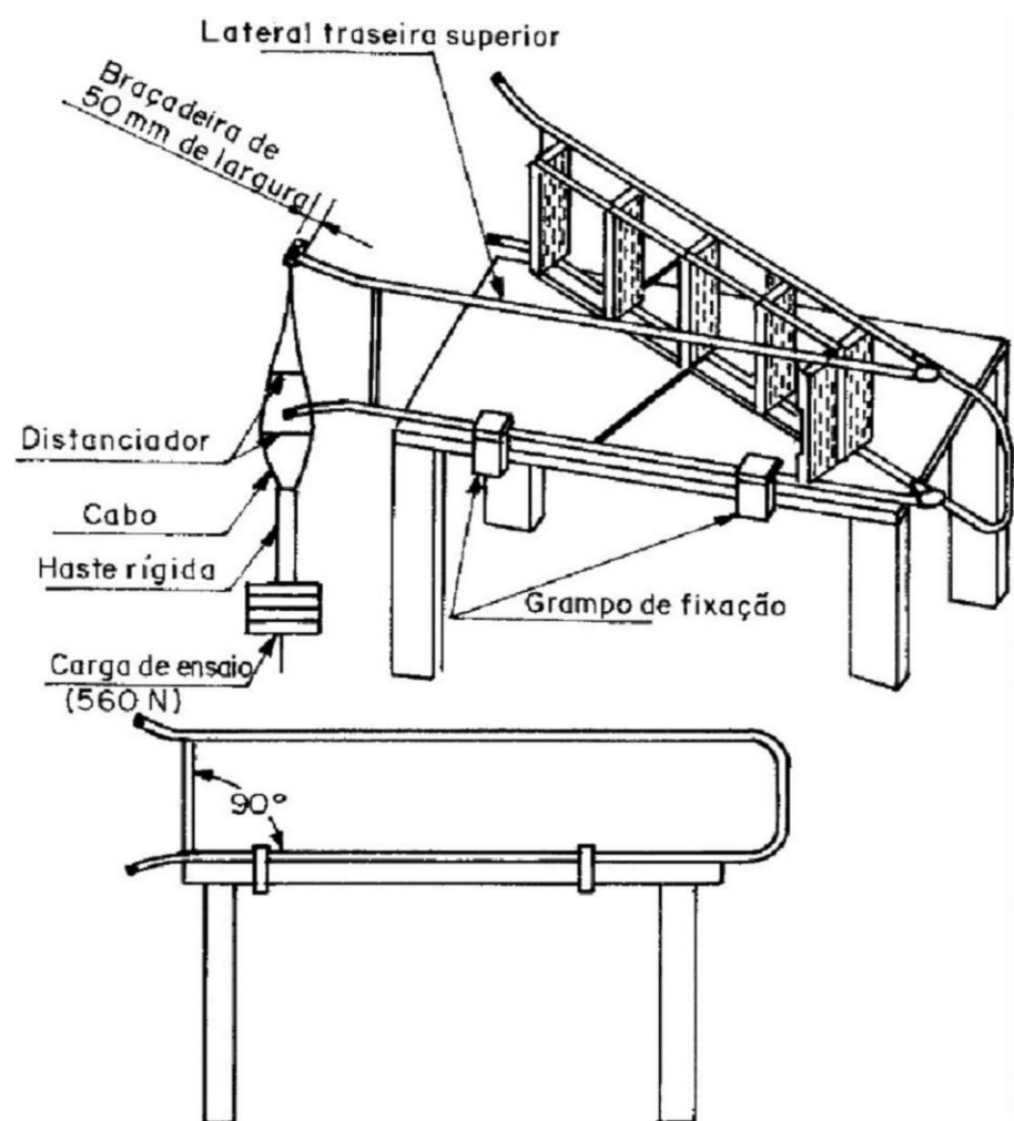
Figura 12 - Ensaio do Balanço Lateral Traseiro - Escadas Convergentes
