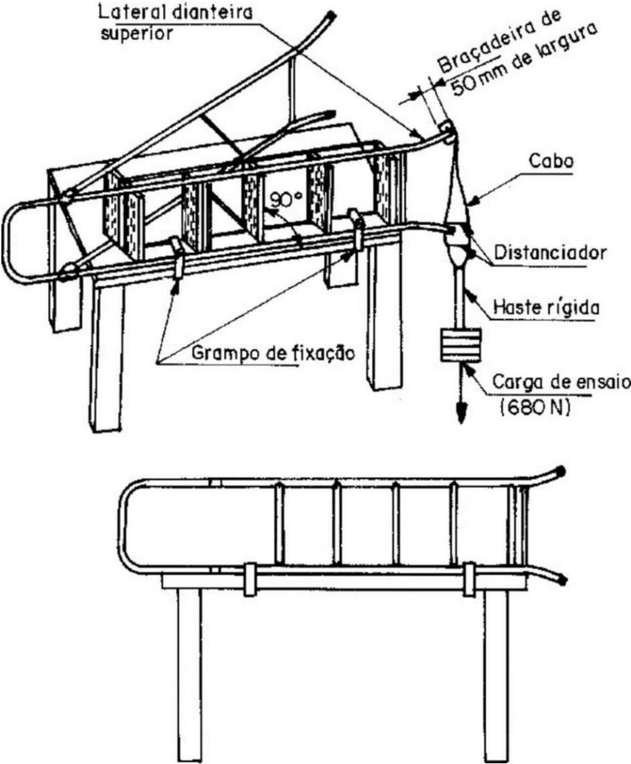
Figura 10 - Ensaio do Balanço Lateral Dianteiro - Escadas Convergentes
