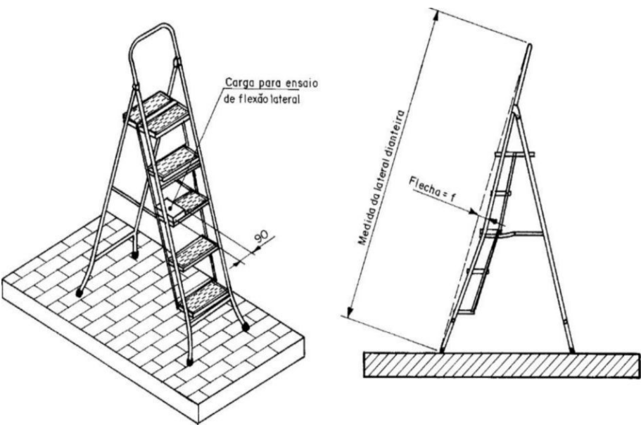
Figura 2 - Ensaio de Flexão do Montante Lateral
