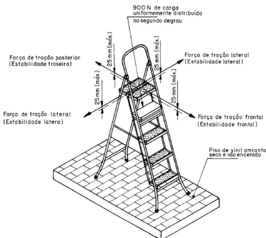
Figura 5 - Ensaio de Estabilidade da Escada
