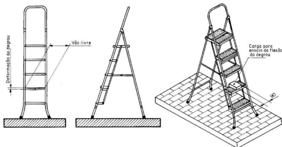
Figura 3 - Ensaio da Flexão do Degrau
