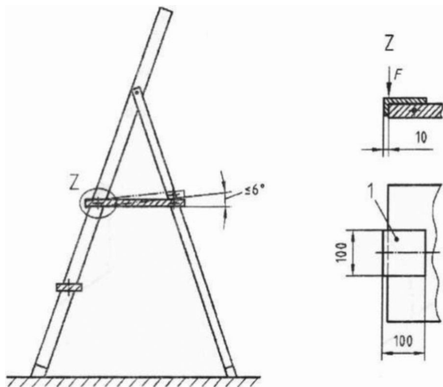
Figura 16 - Ensaio de desengate da plataforma
