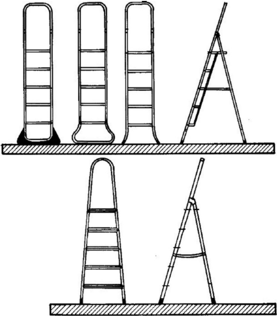
Figura 7 - Escada
