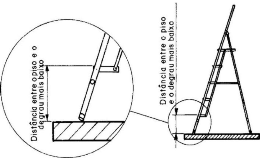
Figura 6 - Distância Entre o Piso e o Degrau Mais Baixo
