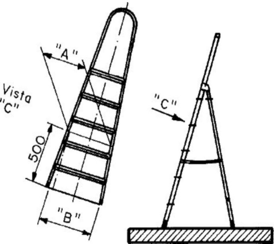
Figura 2 - Convergência da Escada (B-A)
