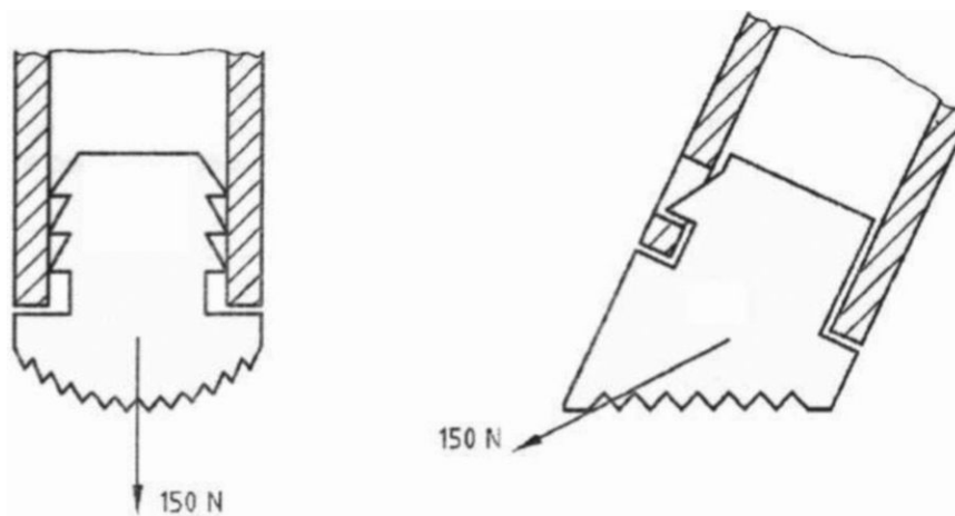
Figura 18 - Ensaio de Tração dos Pés (modelos de sapatas meramente ilustrativas)
