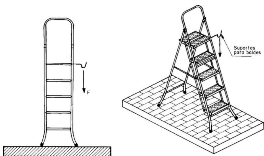
Figura 4 - Ensaio do Suporte para Baldes
