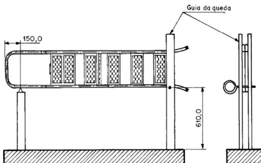
Figura 13 - Queda da Escada
