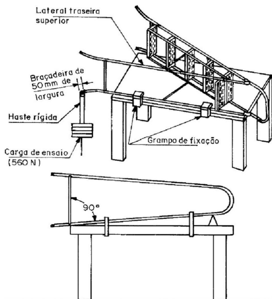
Figura 12 - Ensaio do Balanço Lateral Traseiro - Escadas Convergentes
