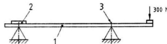
Figura 19 - Ensaio da Alça Superior de Apoio de Pé e Mão
