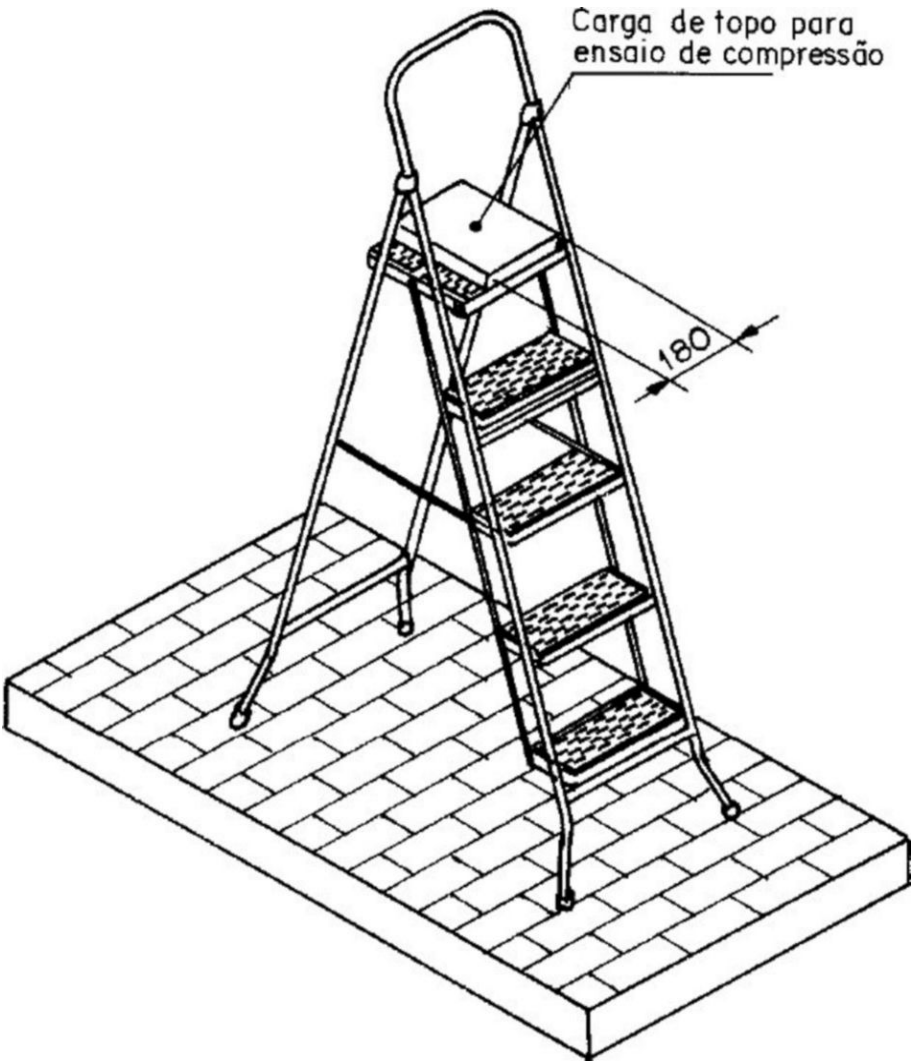
Figura 1 - Ensaio de Compressão
