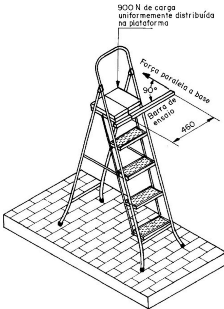
Figura 6 - Ensaio de Estabilidade Torcional
