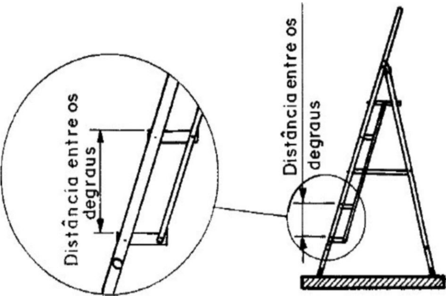
Figura 5 - Distância Entre os Degraus
