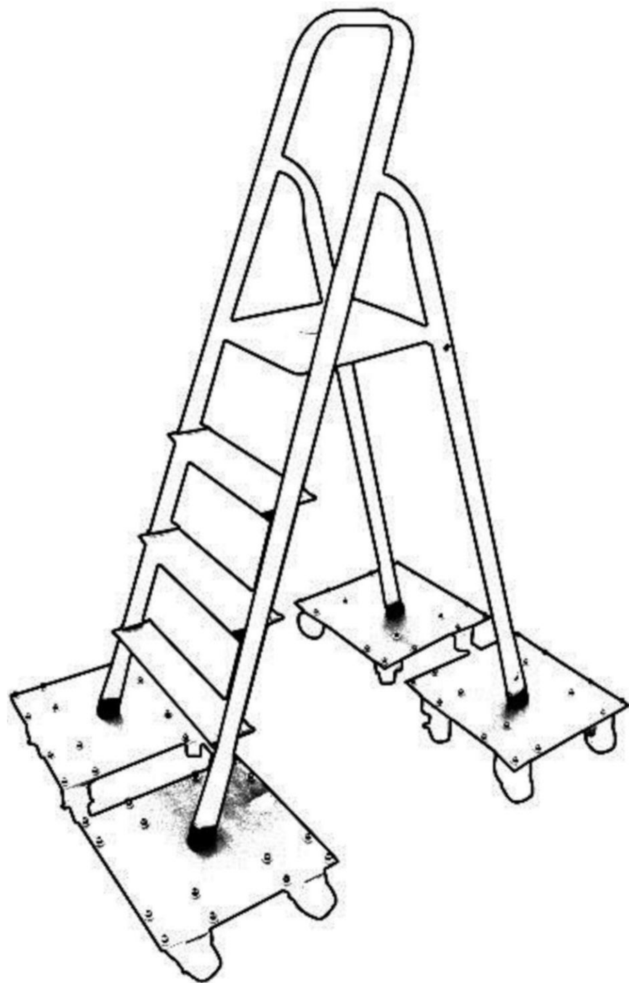
Figura 18 - Ensaio de Tração dos Pés (modelos de sapatas meramente ilustrativas)
