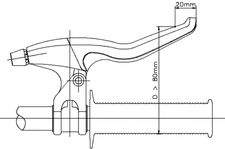
Figura 1 - Exemplo de conjunto de freio de bicicleta de uso adulto.
