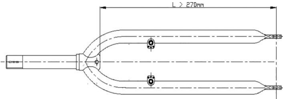
Figura 1 - Dimensões de Garfo Rígido de bicicleta de uso adulto. 4.2 Quadro de Teste Dispositivo utilizado para realização de ensaios, simulando o quadro de bicicleta, quando montado junto ao garfo, com características construtivas adequadas de forma a não interferir nos resultados dos ensaios. 4.3 Família de Garfo de Bicicletas de Uso Adulto Garfos de Bicicletas de Uso Adulto que correspondam às seguintes características, além da definição geral de família de componente de bicicletas estabelecida no subitem 4.1 deste RAC: - Apresentar as mesmas características construtivas, sendo mesmo material das pernas do garfo e mesmo diâmetro externo do canote, conforme item 5 deste Anexo. 5. CLASSIFICAÇÃO DE GARFO EM FAMÍLIA Diferentes modelos de garfo de bicicletas de uso adulto pertencem a uma mesma família quando classificados com uma mesma combinação de cada requisito a seguir:
