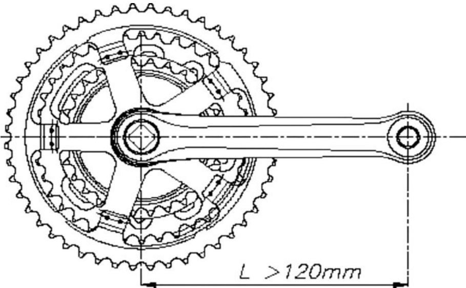
Figura 2 - Dimensões de pedivela montada com engrenagem de bicicleta de uso adulto.
