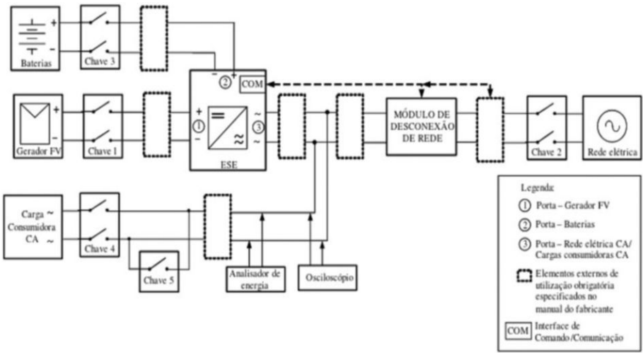
Figura 8 - Diagrama de Ligações para os Ensaios de Inversores On-grid com Bateria de 3 Portas em Operação Ilhada
