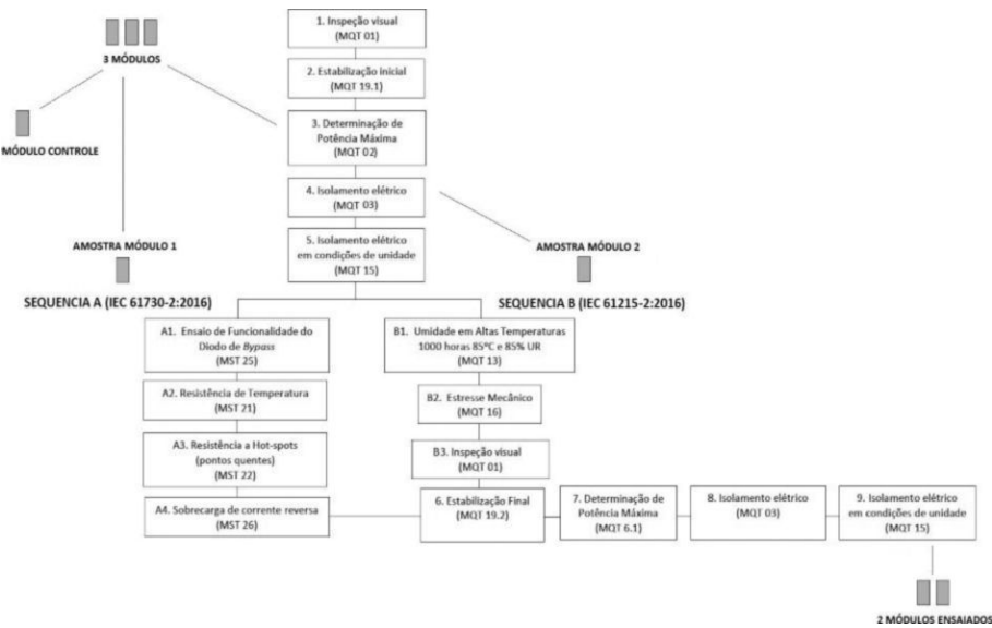
Figura 1 - Fluxograma de Ensaios de Módulos
