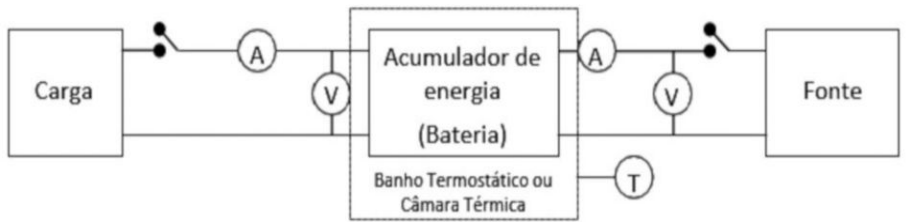
Figura 1 - Configuração dos Aparelhos e Instrumentação para o Ensaio da Capacidade
