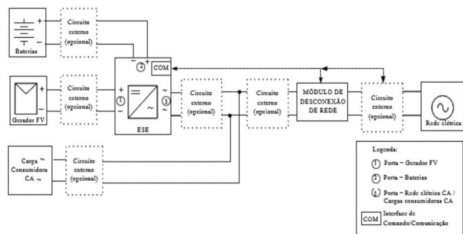
Figura 2 - SFCR com Bateria com Configuração de Inversor de 3 Portas
