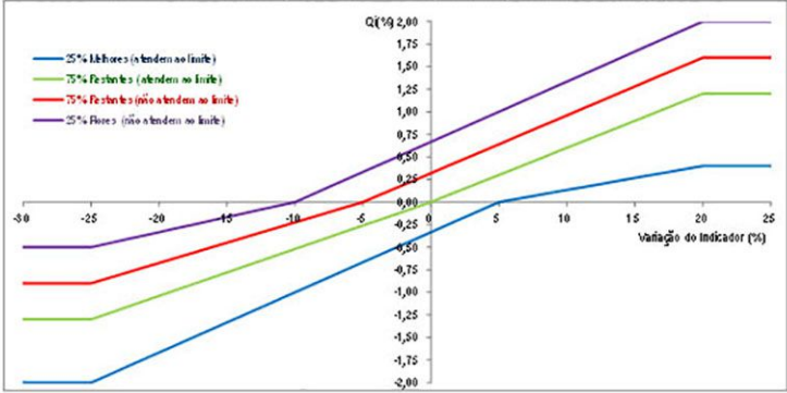
Gráfico II.1 – Curvas para o modelo aplicado para o Indicador DEC
