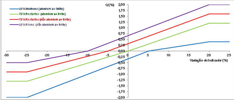
Gráfico II.2 – Curvas para o modelo aplicado para o Indicador FEC
