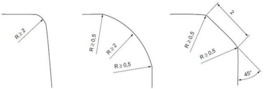
Figura 1 - Exemplos para raios mínimos de bordas e quinas (dimensões em milímetros)
