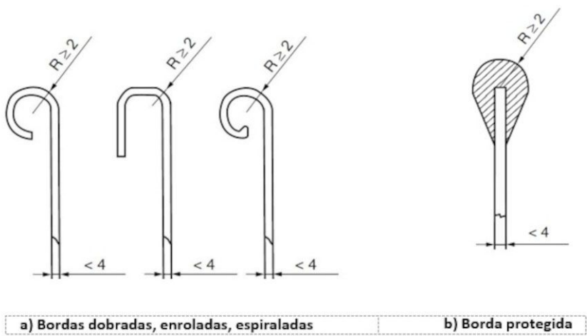
Figura 2 - Bordas enroladas, dobradas, espiraladas e protegidas (Dimensões em milímetros)
