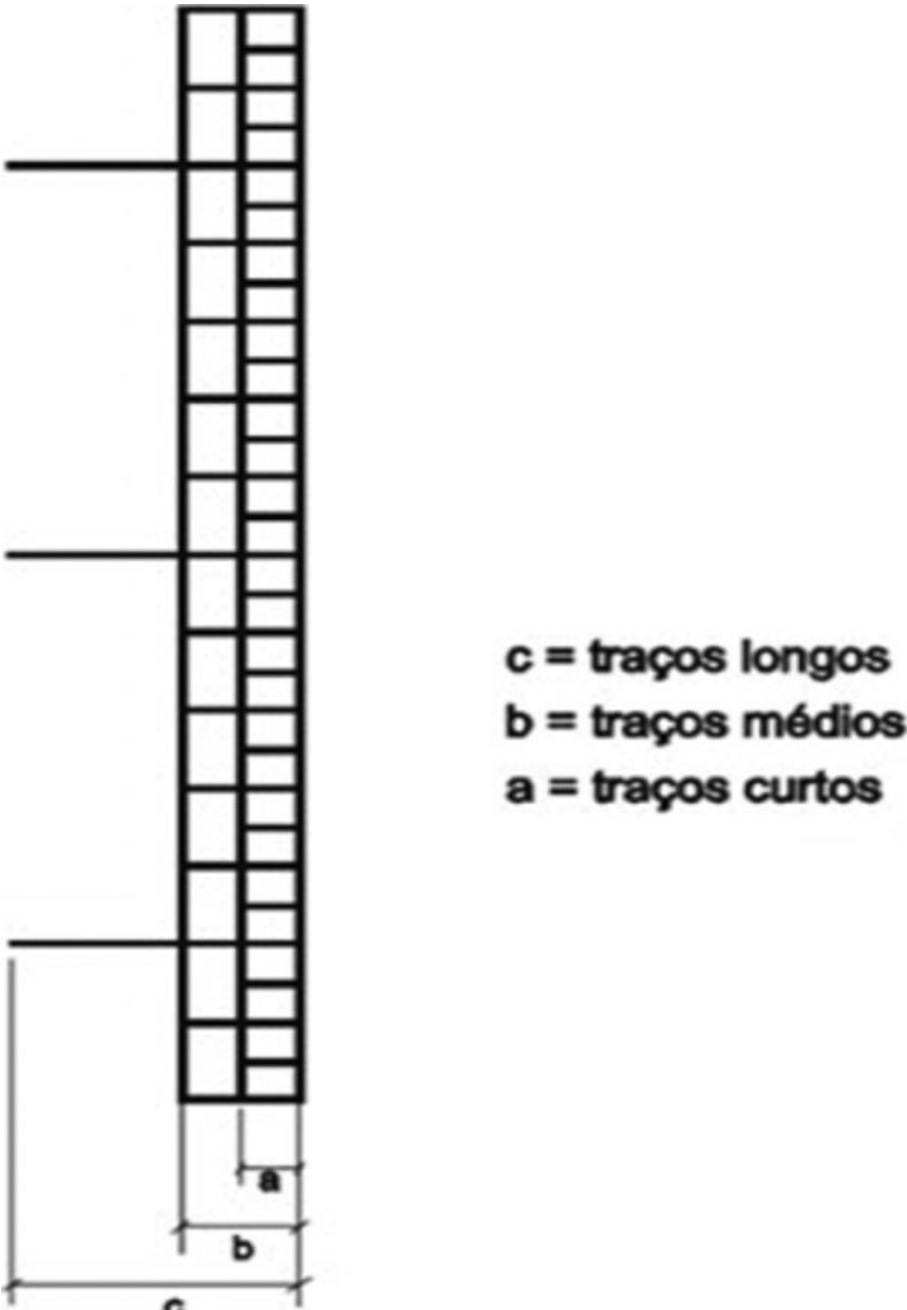
FIGURA 3 - MODELO DE ESCALAS DOS DENSÍMETROS CONFORME SÉRIE
