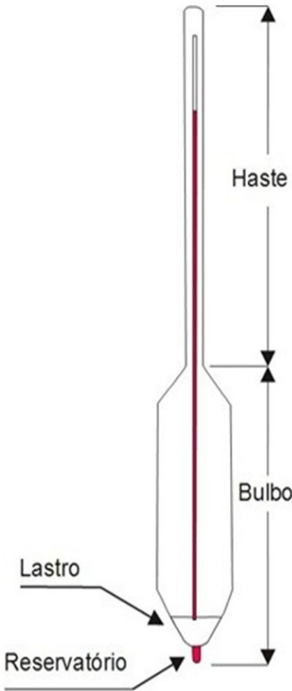
FIGURA 1 - MODELO DE DENSÍMETRO TERMOCOMPENSADO
