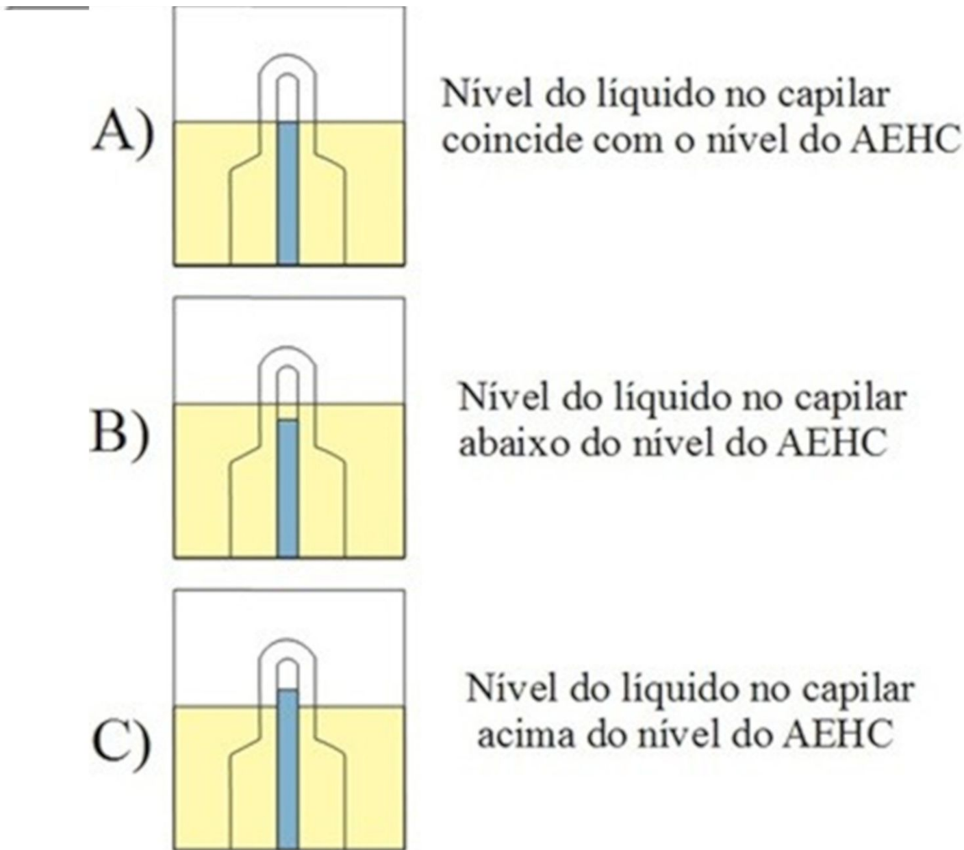
FIGURA 2 - NÍVEL DO LÍQUIDO CAPILAR EM RELAÇÃO AO EHC
