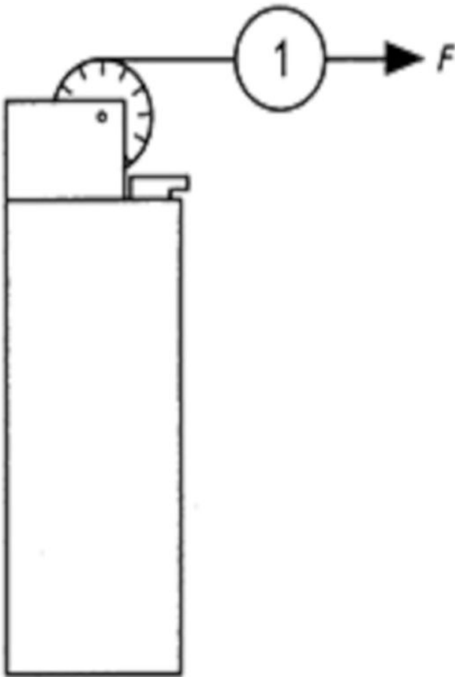
Legenda: F Geração de chama por força atuante 1 Medidor de força Figura 2 - Aplicação de força atuante de geração de chama - Atuador rotativo 3.2 A altura da chama do isqueiro deve atender o seguinte: a) Os isqueiros não ajustáveis, postmixing e premixing, não podem ser capazes de produzir uma altura de chama maior que 50 mm. b) Os isqueiros postmixing ajustáveis devem ter a altura da chama ajustada pelo fabricante, de forma que o isqueiro, quando aceso pela primeira vez pelo usuário - sem mudança do ajuste - não produza uma altura de chama maior que 100 mm.
