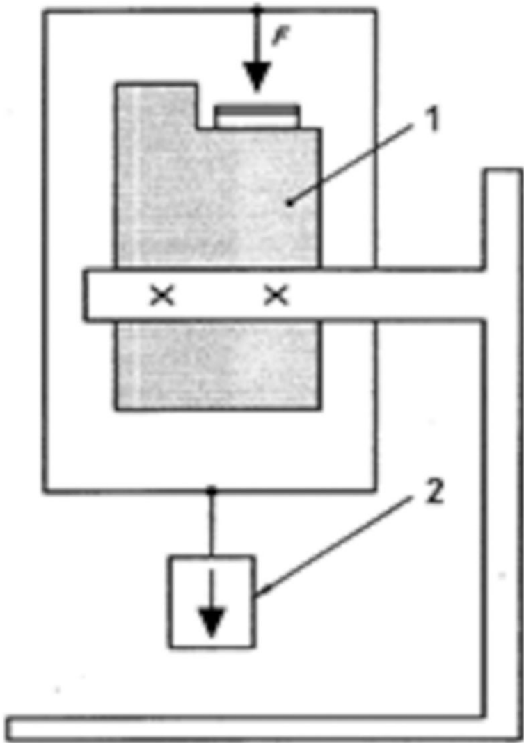
Legenda: F Geração de chama por força atuante 1 Isqueiro 2 Massa Figura 1 - Aplicação de força atuante de geração de chama - Botão de empurrar acionador
