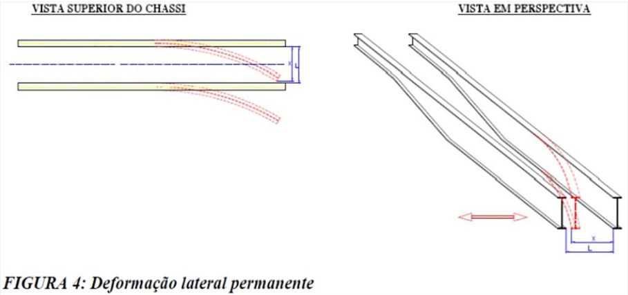
FIGURA 4: Deformação lateral permanente
