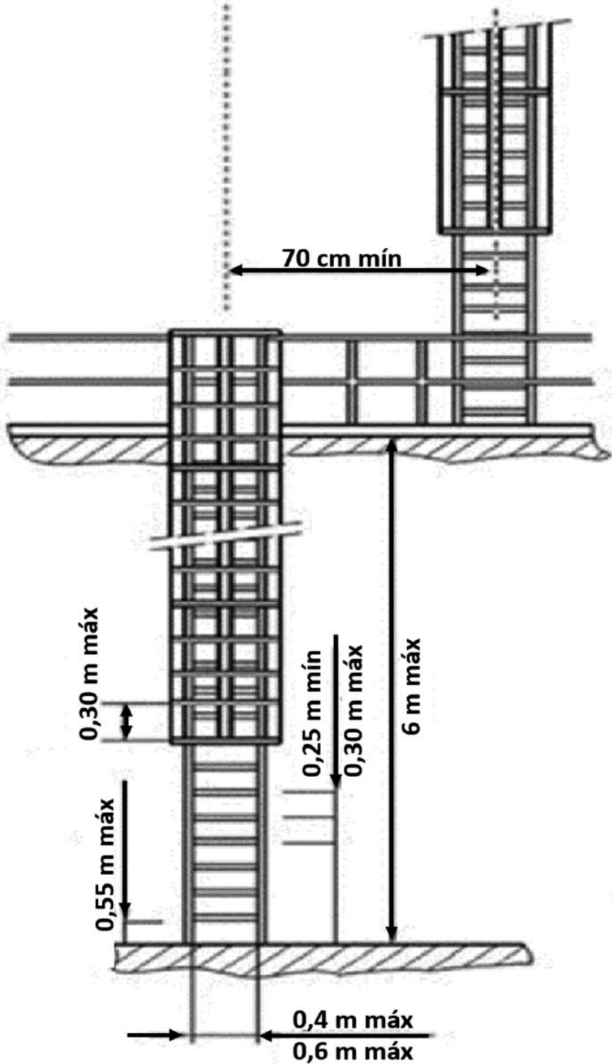
Figura 3: Exemplo de escada fixa do tipo marinheiro
