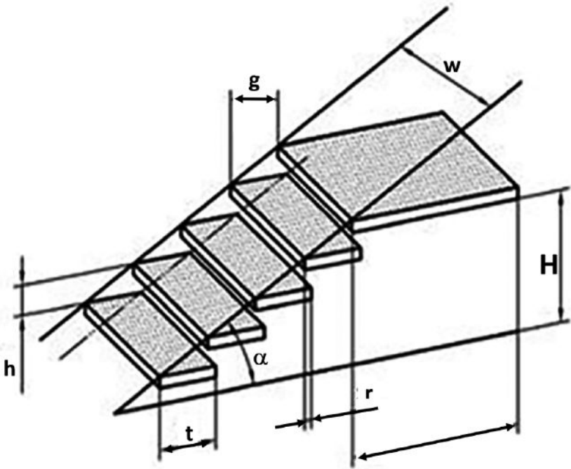
Figura 2: Exemplo de escada sem espelho
