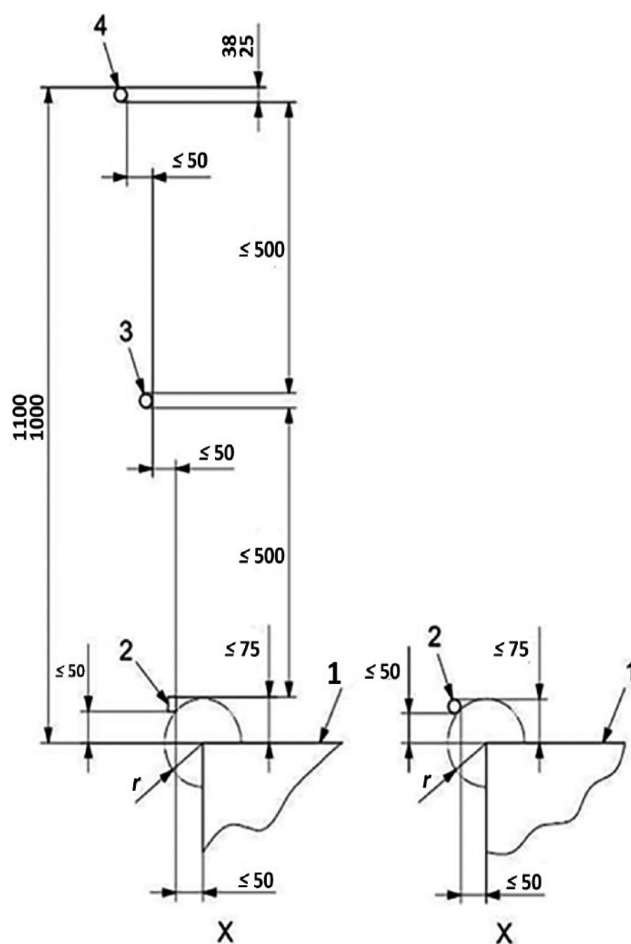
Figura 5: Sistema de proteção contra quedas em plataforma (dimensões em milímetros)
