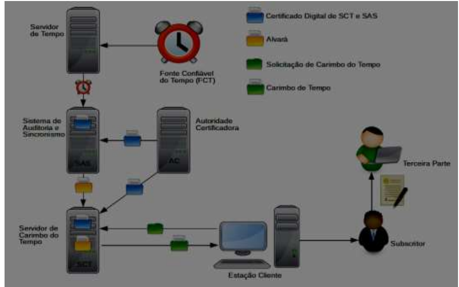
Figura 1 - Modelo de Funcionamento do Carimbo do Tempo da ICP-Brasil.
