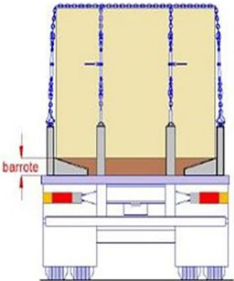
Amarração do bloco de rocha convencional:
