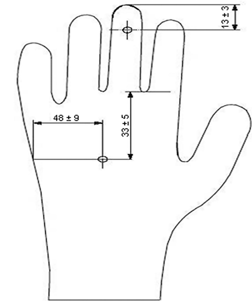
Figura A.2 - Pontos de medição para espessura da luva Nota: A distância de 48 mm ± 9 mm localiza o centro aproximado da palma para luvas de tamanhos diferentes.
