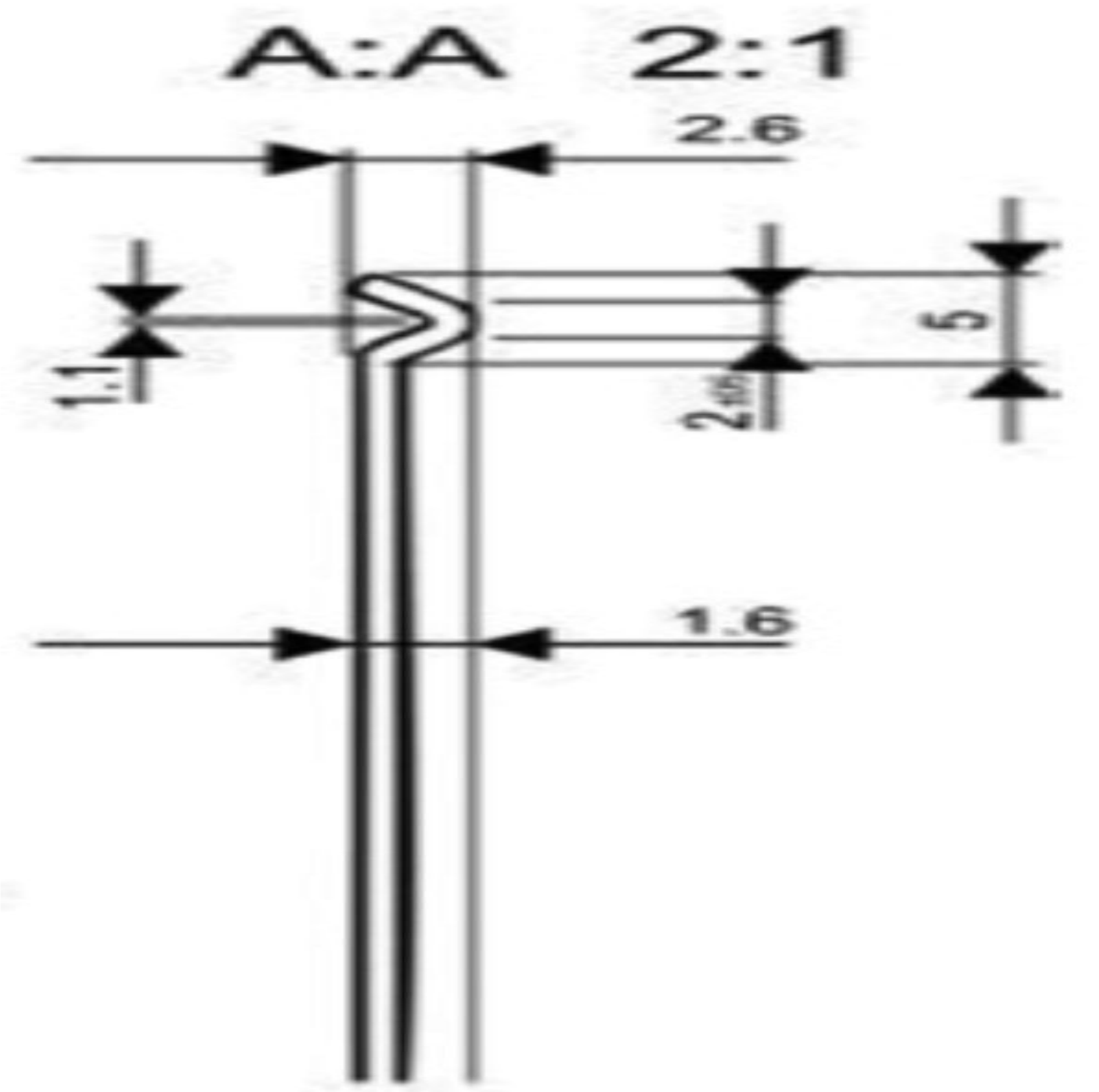
FIGURA II - PLACA DEMAIS VEÍCULOS
