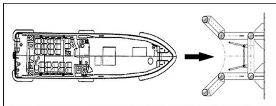
Figura 2 - Vista superior do sistema composto por lancha do tipo surfer e atracadouro.
