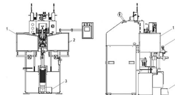
Figura 21: Máquina de alta frequência com mesa móvel manual
