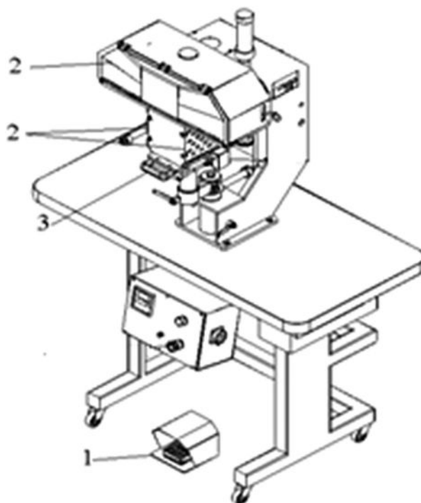
Figura 30: Máquina de carimbar solas e palmilhas
