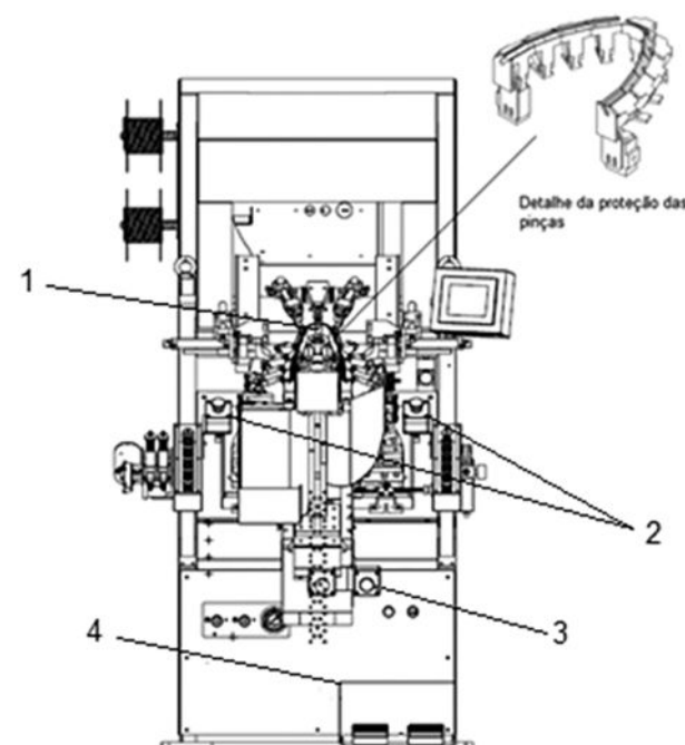
Figura 17: Máquina de montar bicos
