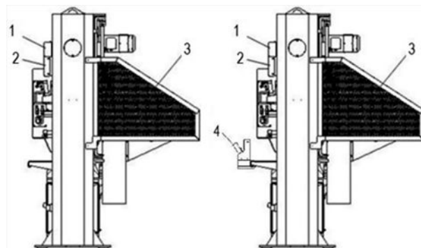
Figura 5: Balancim tipo ponte manual - Vista lateral
