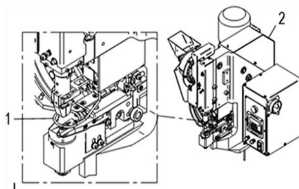
Figura 10: Máquina automática de aplicar ilhós, rebites e adornos - detalhe da vista frontal
