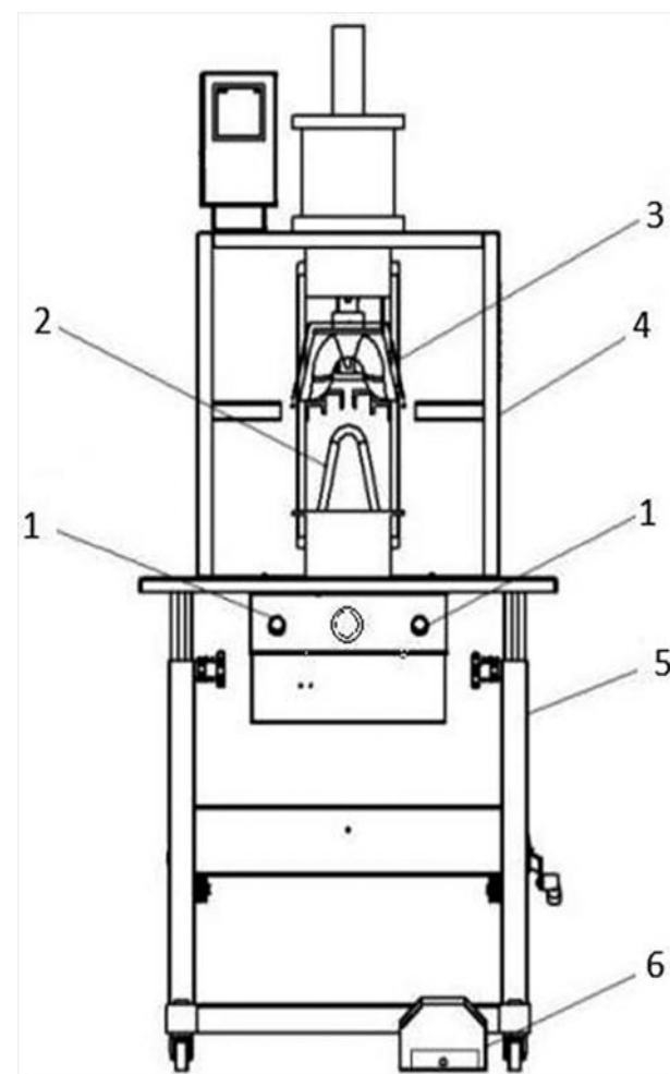
Figura 7: Máquina de cambrê com borrachão - Vista Frontal
