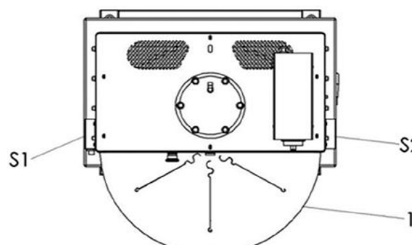
Figura 16: Máquina de prato rotativo (dublar) - vista superior
