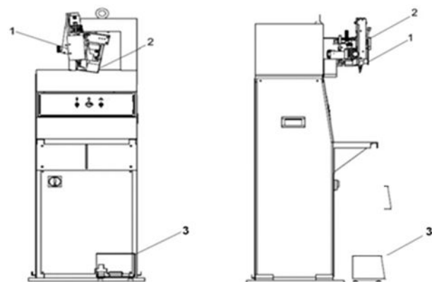
Figura 29: Máquina de montar lados - Vista frontal e lateral
