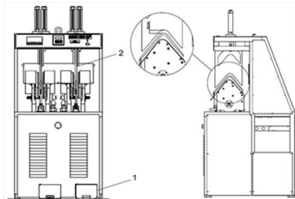
Figura 8: Máquina de cambrê facão - Vista frontal
