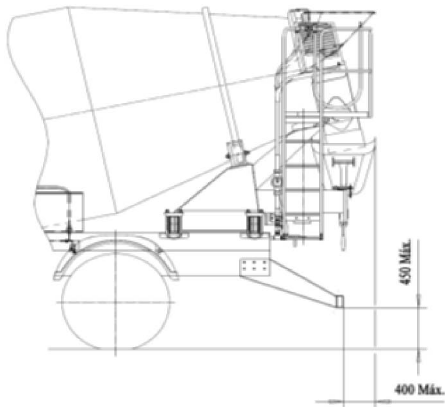
Figura 3a - Vista lateral da parte traseira dos veículos - Betoneira
