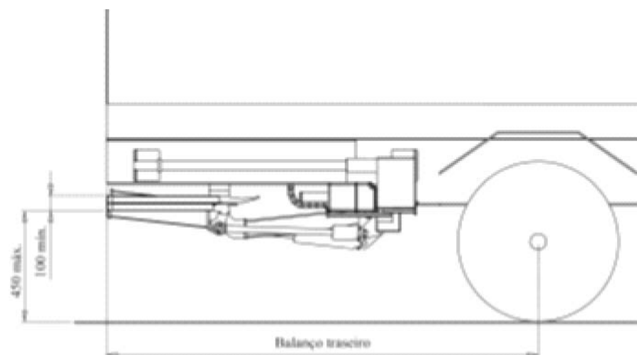
Figura 4 - Exemplos de para-choque de veículo equipado com plataforma elevatória
