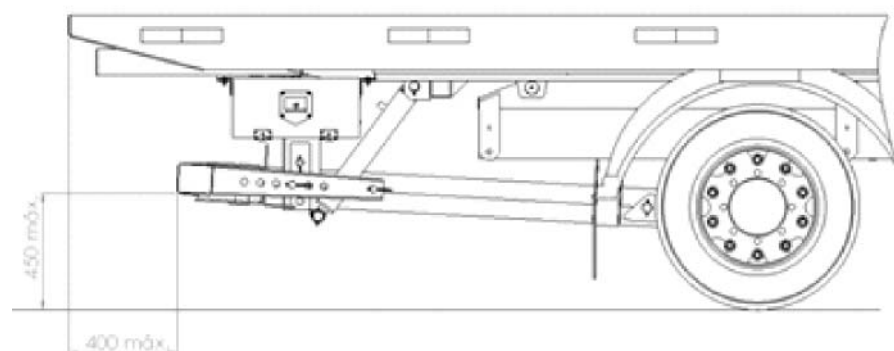
Figura 3b - Vista lateral da parte traseira dos veículos - Plataforma autossocorro com Asa Delta
