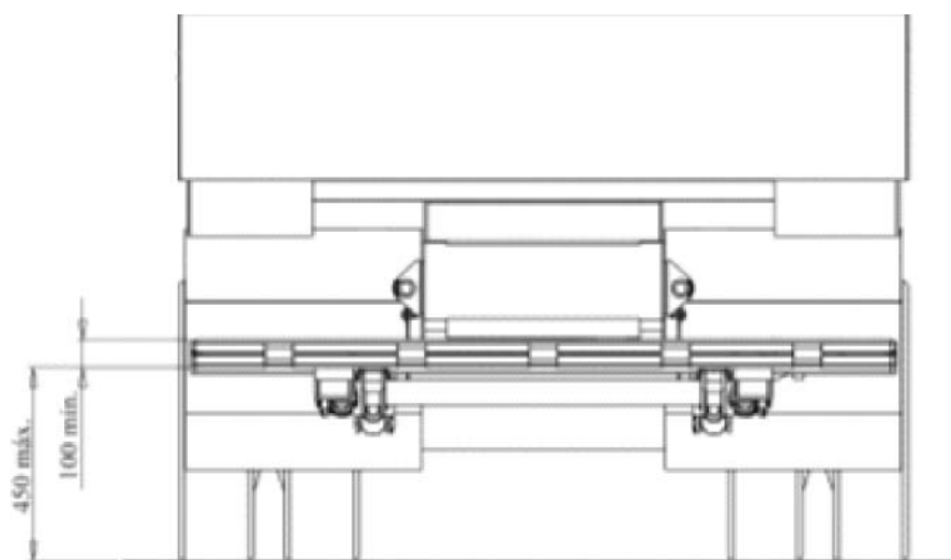
Figura 5 - Plataforma elevatória com a função de para-choque
