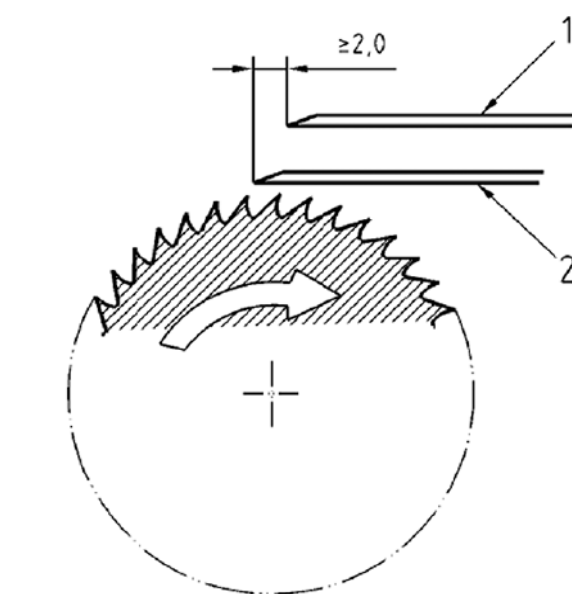
Figura 9 - Detalhe das zonas de perigo 1, 2 e 3 da máquina aberta de descourear e retirar a pele e a membrana (com pente raspador)
