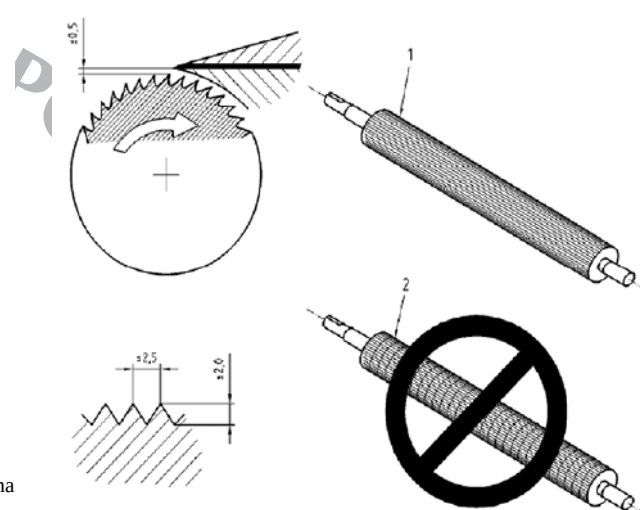
Figura 12 - Requisitos de segurança do cilindro de arraste
