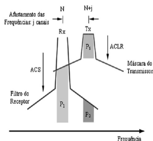
Figura 1 - Sistema transmissor e receptor sem filtragem adicional.
