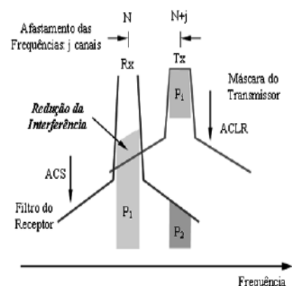
Figura 2 - Redução da interferência por adição de filtro na transmissão.
