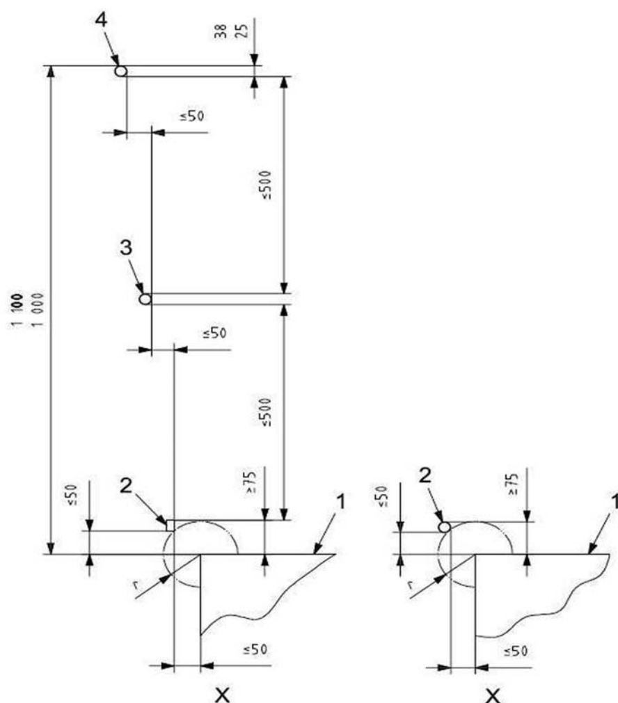
Figura 5: Sistema de proteção contra quedas em plataforma. (dimensões em milímetros)
