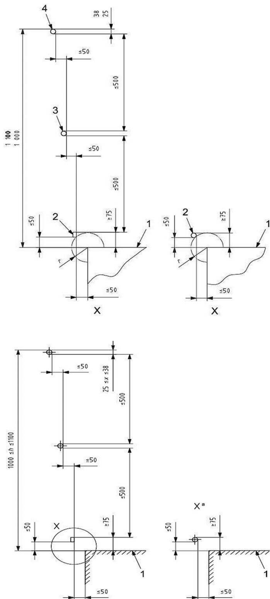
Figura 5: Sistema de proteção contra quedas em plataforma. (dimensões em milímetros)
