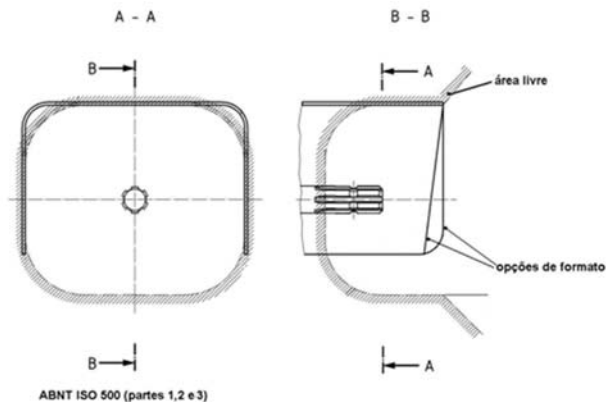
QUADROS E FIGURAS AUXILIARES Figura 1 - Cobertura de proteção da TDP para tratores agrí- colas
