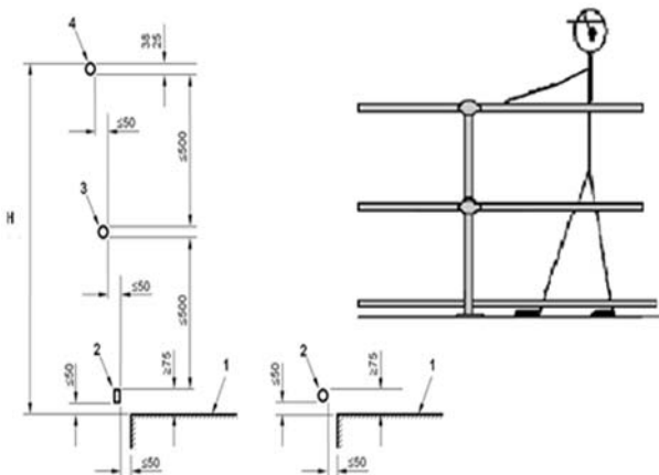
Figura 5: Sistema de proteção contra quedas em plataforma. (dimensões em milímetros)
