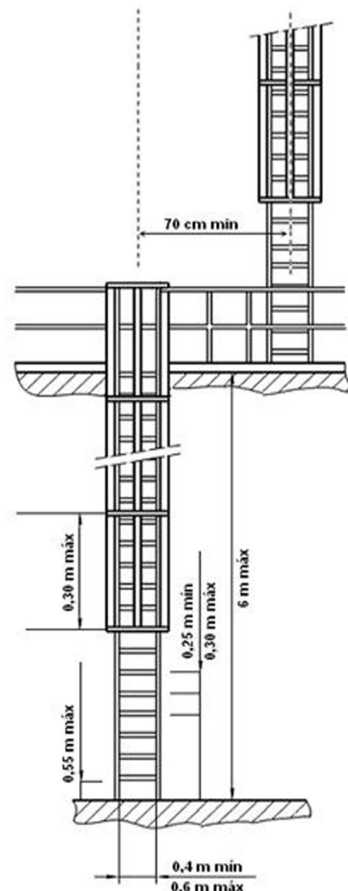
Figura 3: Exemplo de escada fixa do tipo marinho.
