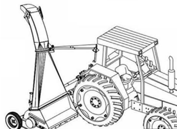
Forrageira tracionada: implemento agrícola que, quando acoplado a um trator agrícola, pode realizar a operação de colheita ou recolhimento e trituração da planta forrageira, sendo o material triturado, como forragem, depositado em contentores ou veículos separados de transbordo.
