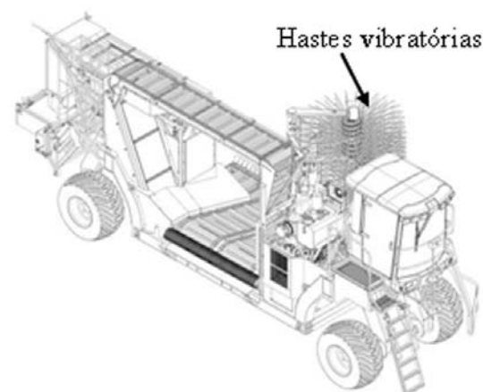
Colhedora de laranja: máquina agrícola autopropelida que efetua a colheita da laranja e outros cítricos similares.
