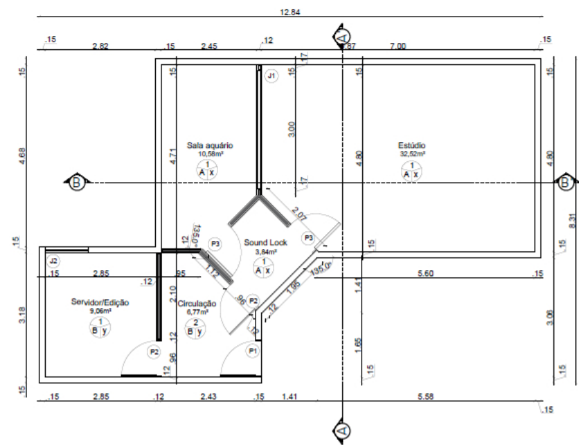
Planta Baixa - Especificações Escala 1/50
