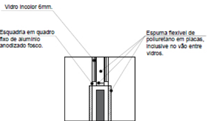
Detalhe 01 Escala 1/10
