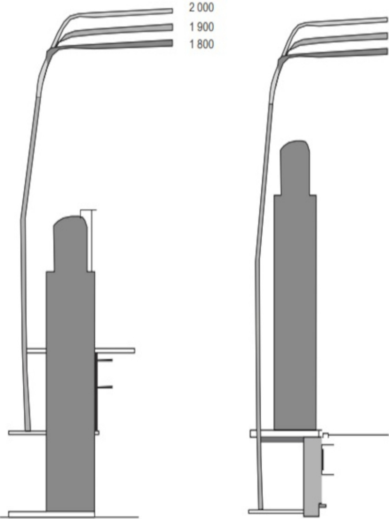
Figura 3- Deslocamento vertical do gabarito (dimensões em mm).
