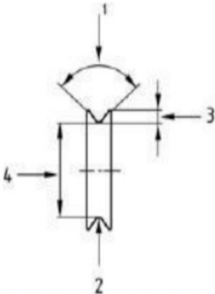
Figura C.1 - Dimensões e ângulo dos canais da polia.
