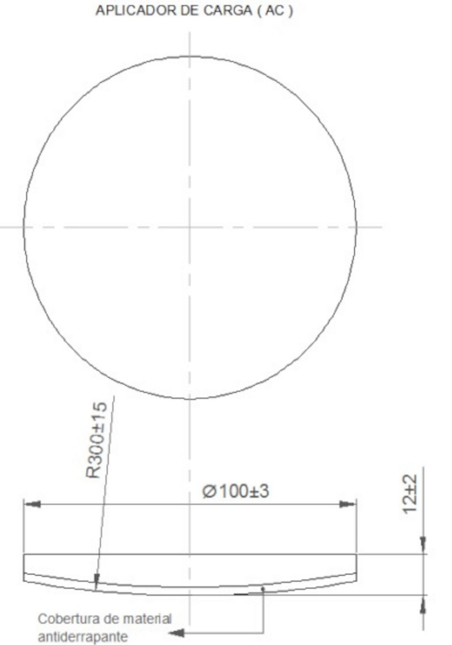
Figura I.1 - Aplicador de Carga (AC)
