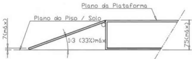
Figura 7 - Características da rampa da plataforma elevatória veicular (dimensões em mm).
