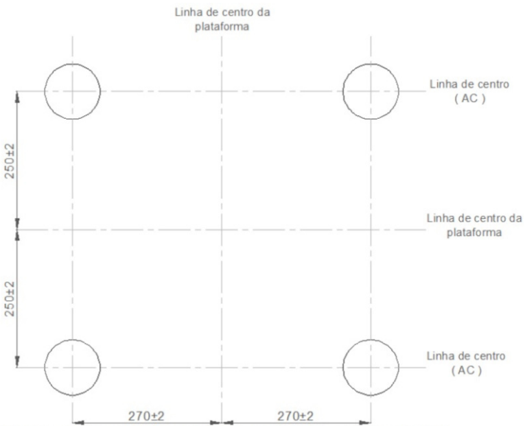
Figura I.2 - Configuração dos Dispositivos de Aplicação de Carga (AC)
