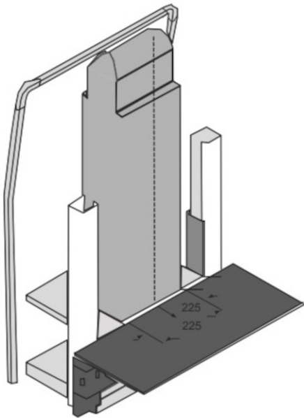
Figura 4 - Representação tridimensional do gabarito (dimensões em mm).
