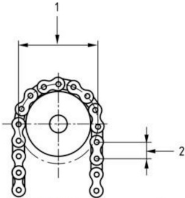
Figura C.4 - Círculo divisório/primitivo para correntes de aço
