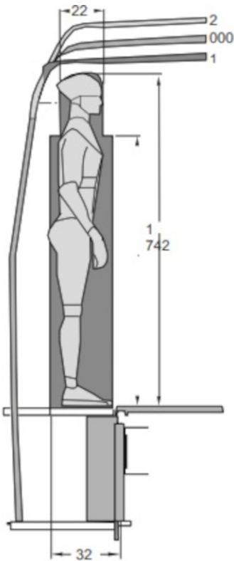
Figura 2 - Vista lateral da área do gabarito (dimensões em mm).
