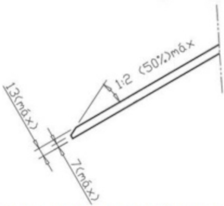
Figura 8 - Borda frontal da rampa (dimensões em mm).
