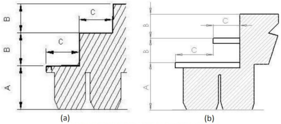
Figuras 6 (a) e (b) - Degraus das escadas.
