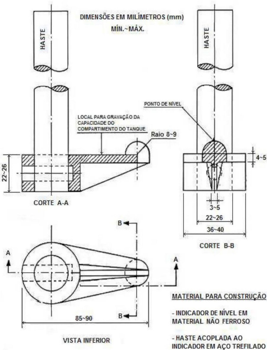
Anexo 4 - Forma de fixação de dispositivo de referência para múltiplos níveis
