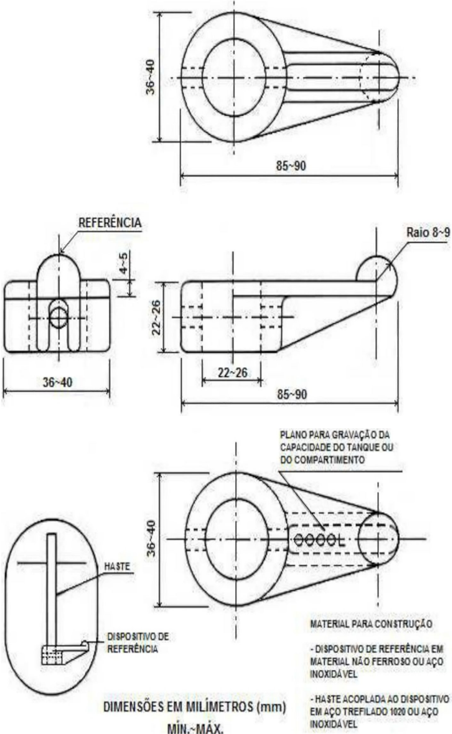
Anexo 2 - Modelo de dispositivo de referência (modelo A)
